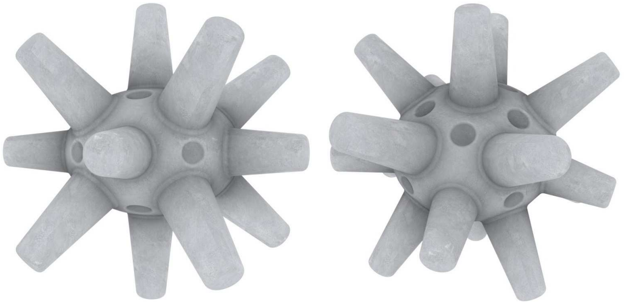
fig. 1 - Masso artificiale RICCIO in ecocemento a ph basico, con inerti di riciclo da C&D e fibra di Posidonia oceanica
