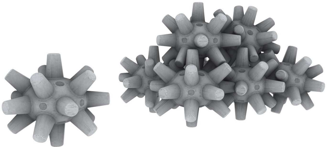
fig. 2 - Scogliera (emersa o sommersa) realizzata con massi artificiali RICCIO: elevato interlocking masso-masso
