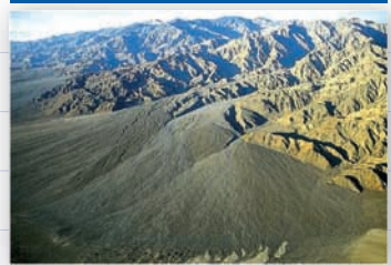
I conoidi alluvionali Alluvial fans
